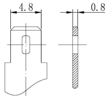
Позиция клемм
